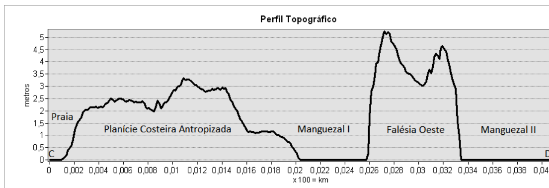
Figura 5: Perfil topográfico CD em Salinópolis, demonstrando grande extensão compondo a Zona Costeira de Baixa Elevação ao longo dos setores costeiros.
